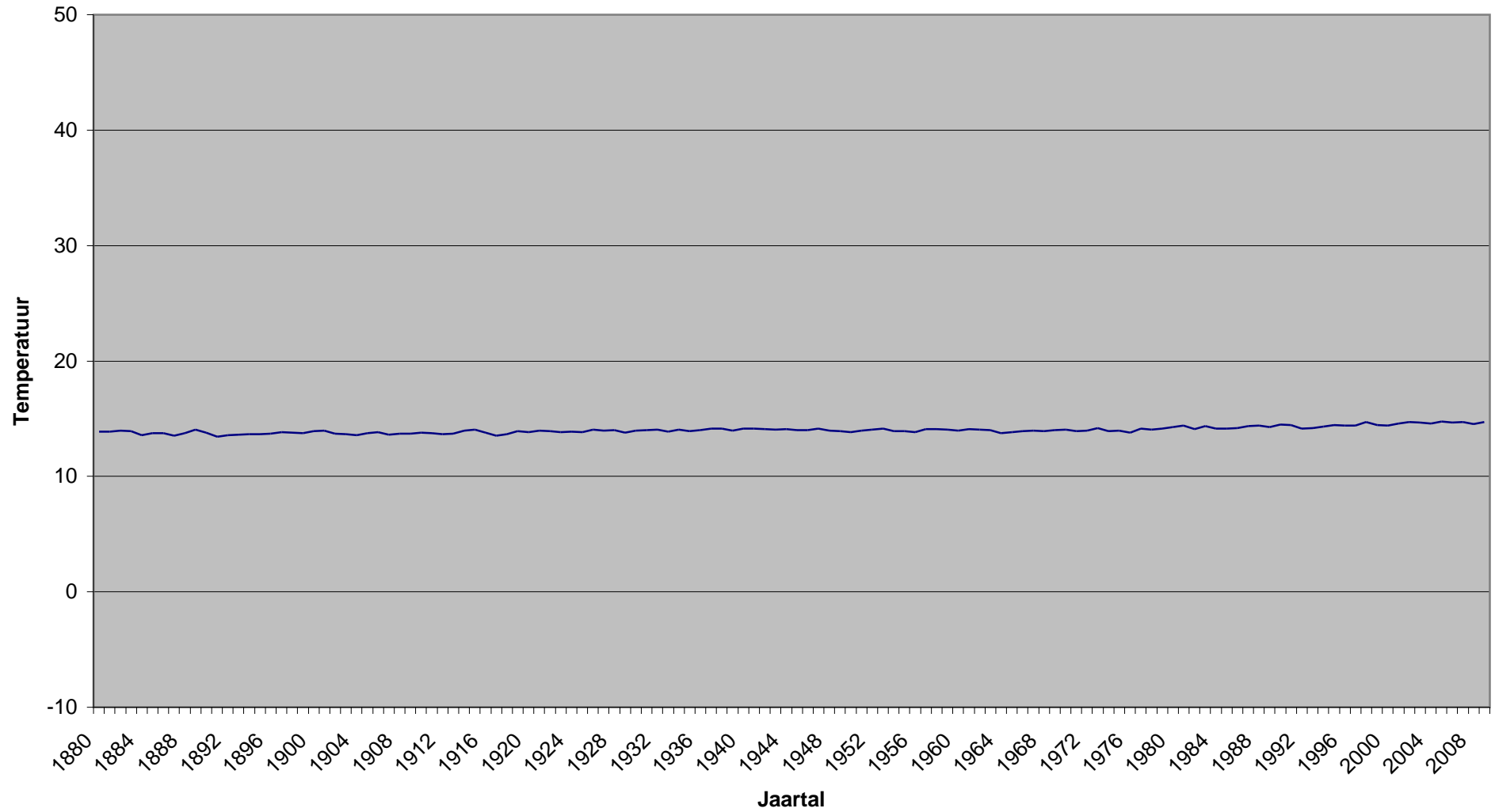
Aardtemperaturen 1880-2009 (www.frankdeboosere.be) met normale temperatuur-X-AS !!
